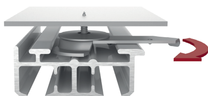
Twist beslag
